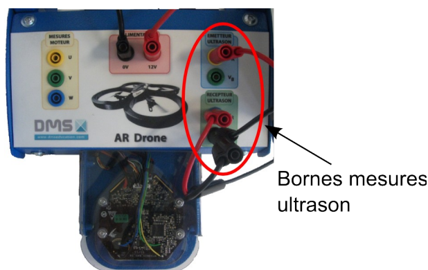
Fig. 118: Mesures altimètre à ultrason
